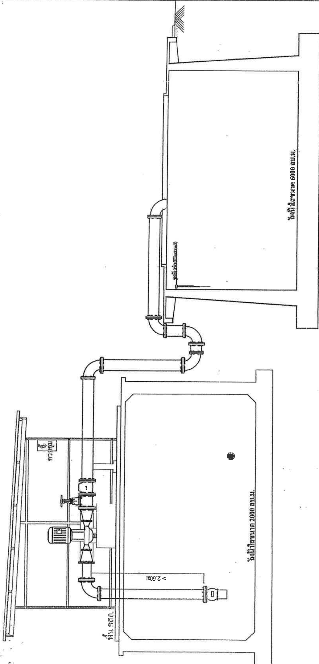
รูปตัดแสดงการประสานท่อและอุปกรณ์จากโรงสูบน้ำจนถึงน้ำใส 2000ลิตร.ม. ไปยังบนฝาปิดถังน้ำใส 6000ลิตร.ม.
